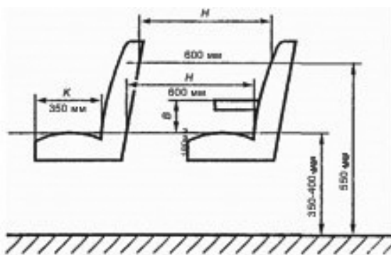
Зураг 2. Суудлын байрлалын хэмжээ (Жишээ зураг)
