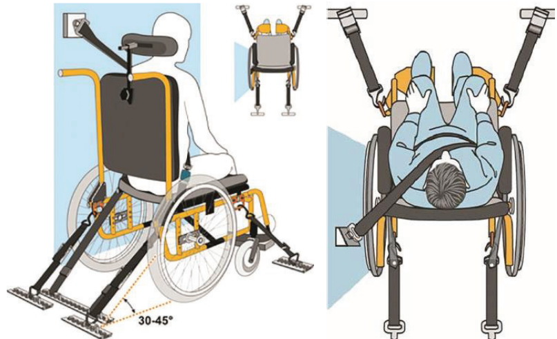
Зураг 7. Автобусанд тэргэнцрийг түгжсэн байдал (Жишээ зураг)
